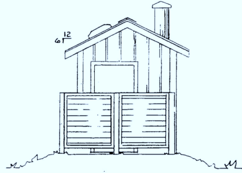
RIGHT ELEVATION Scale: 1/4" = 1'-0"
