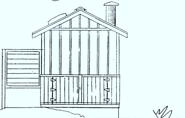
RIGHT ELEVATION SCALE: 1/4" = 1'-0"
